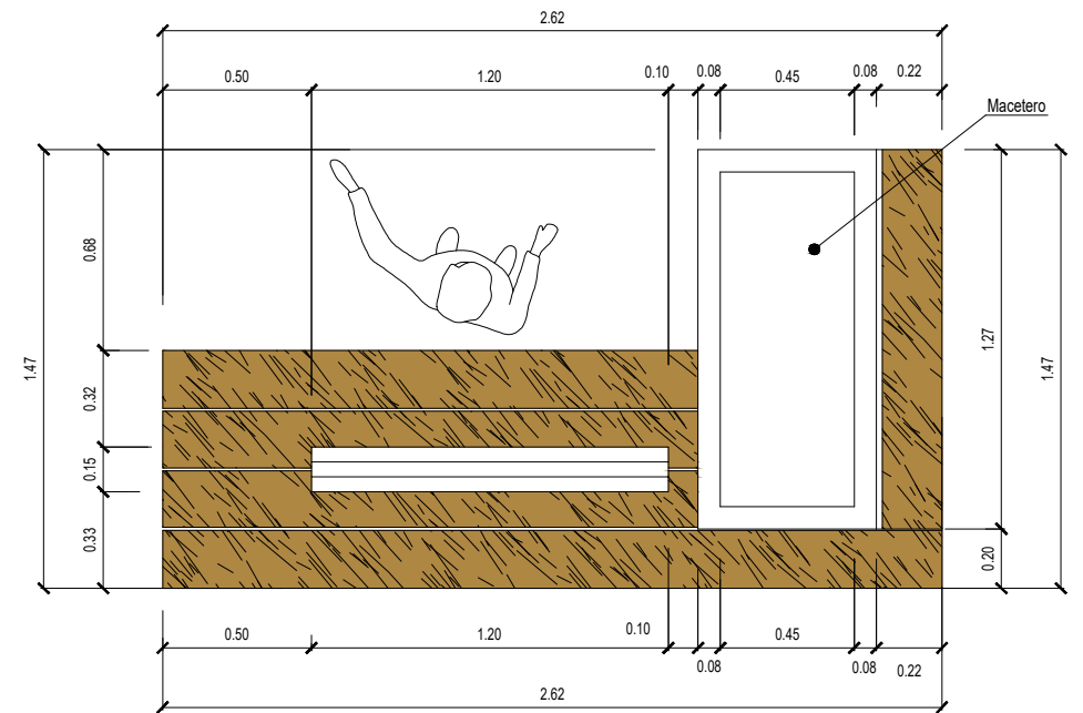
ESCAÑO N°3 PLANTA ARQUITECTURA
