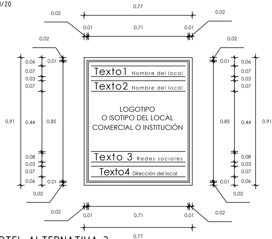
CARTEL ALTERNATIVA 3 ESCALA 1/20
