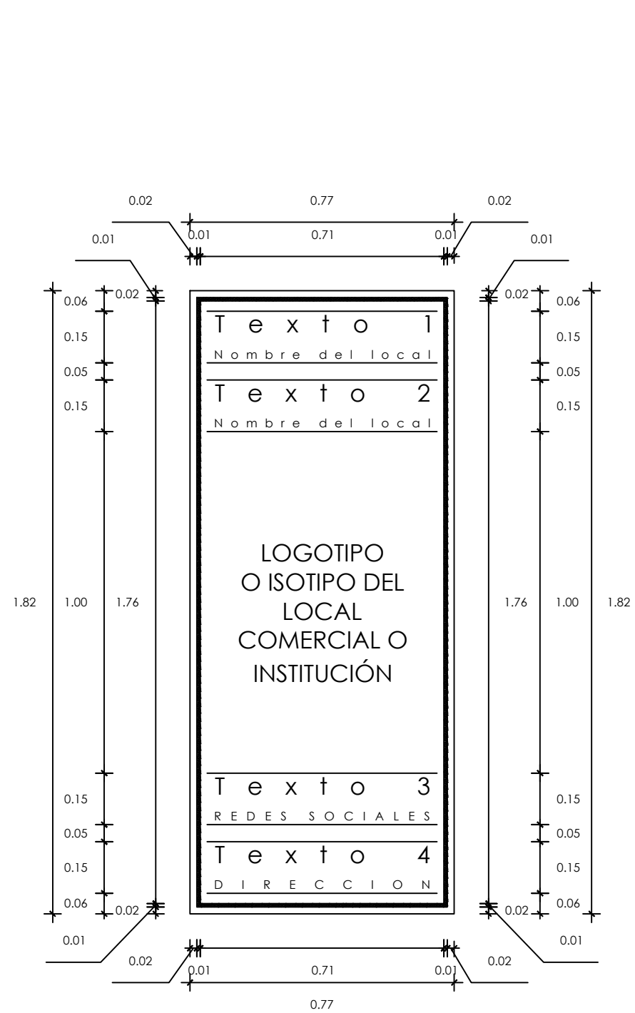
CARTEL ALTERNATIVA 1 ESCALA 1/20
