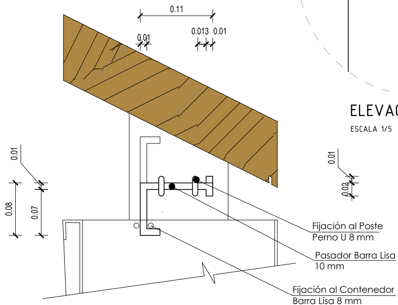
ELEVACIÓN LATERAL DETALLE BASURERO 1
