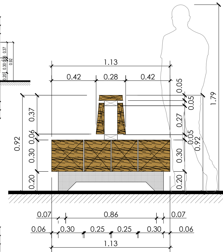
ESCAÑO N°1 CORTE TRANSVERSAL
