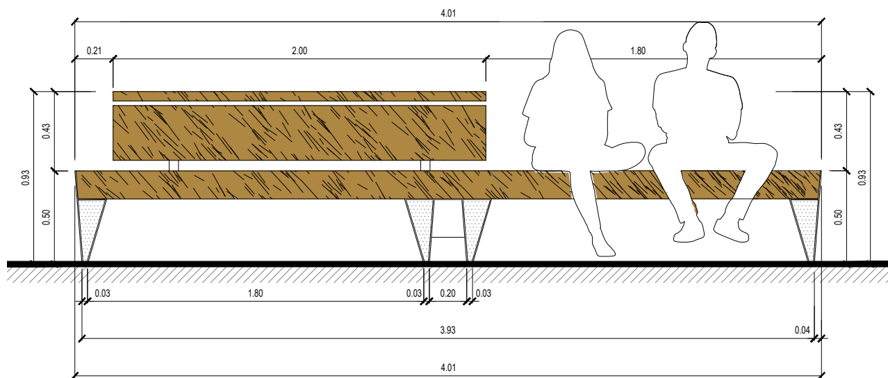
ESCAÑO N°4 ALZADO FRONTAL
