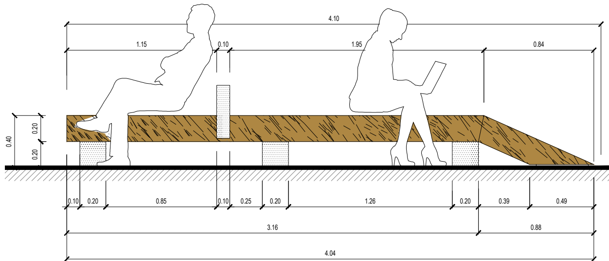
ESCAÑO N°5 ALZADO FRONTAL
