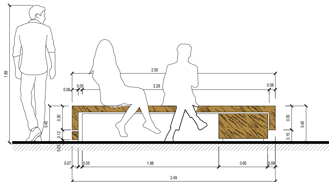
ESCAÑO N°6 ALZADO LATERAL
