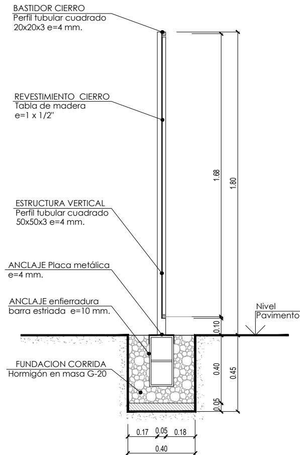
CORTE TRANSVERSAL ALTERNATIVA 3
