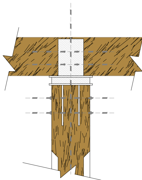
Alzado frontal Capitel Alternativa N°1. Escala 1/10
