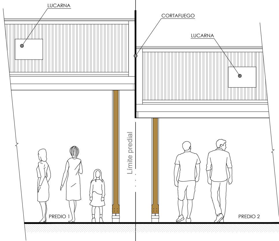
DETALLE ENCUENTRO ENTRE VEREDAS CUBIERTAS EN DISTINTO NIVEL SIN ESCALA
