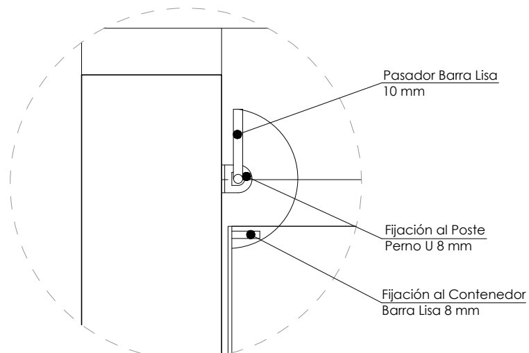
ELEVACIÓN FRONTAL DETALLE BASURERO 1
