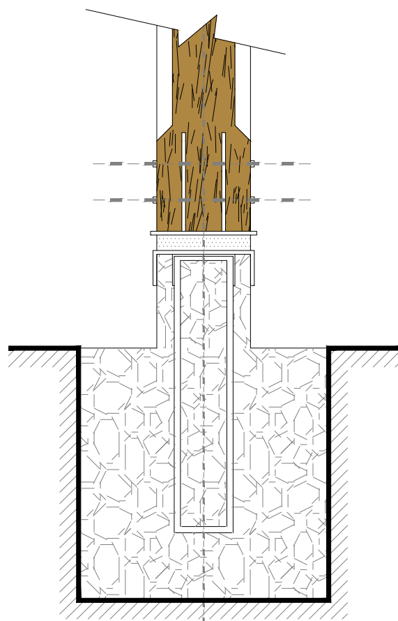
Alzado frontal Base alternativa 2
