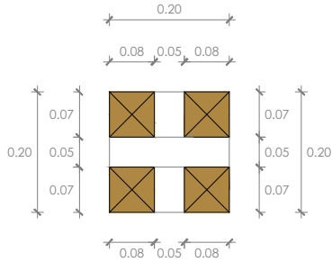
Planta Pilar armado alternativa 1
