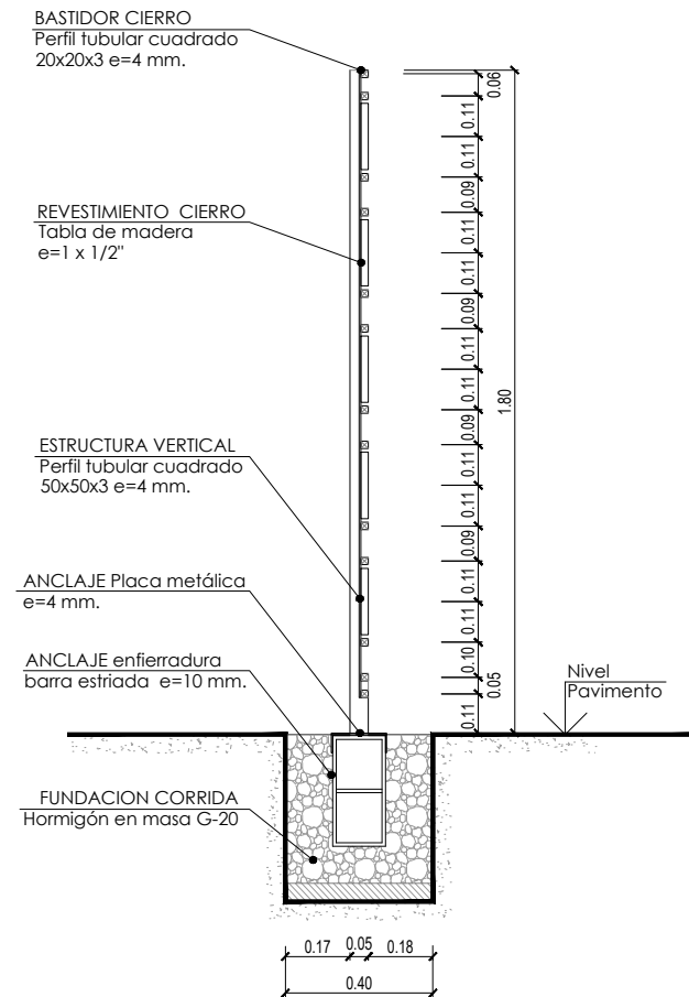
CORTE TRANSVERSAL ALTERNATIVA 5
