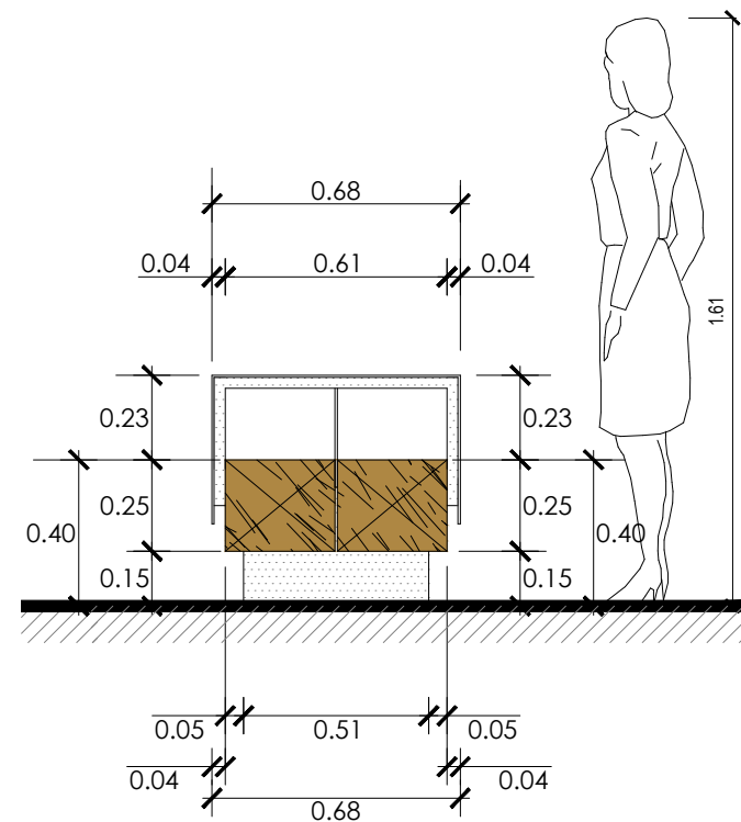
ESCAÑO N°7 CORTE TRANSVERSAL
