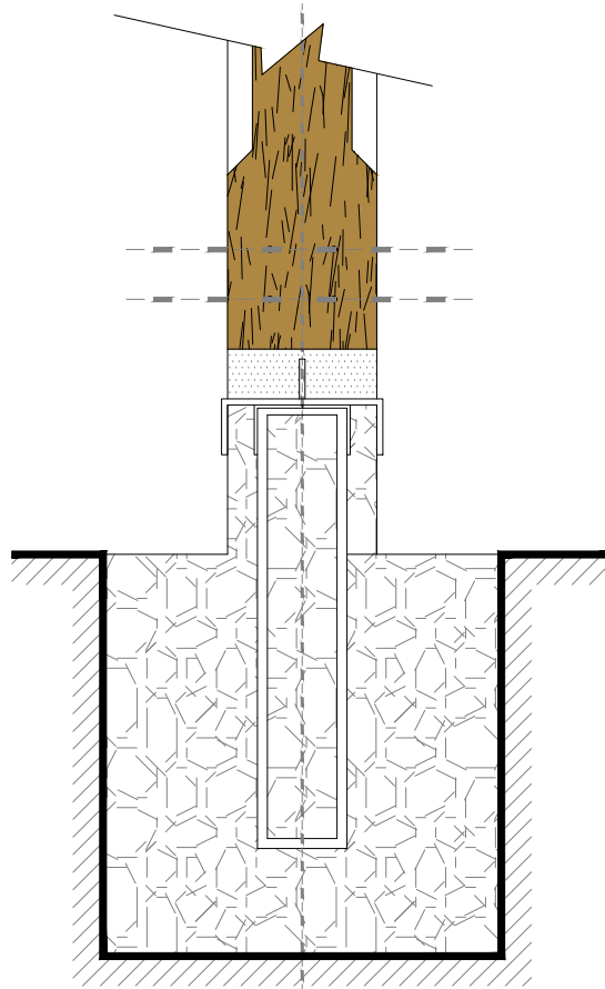
Alzado frontal Base alternativa 1
