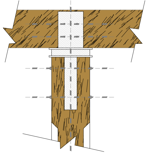
Alzado frontal capitel alternativa 3
