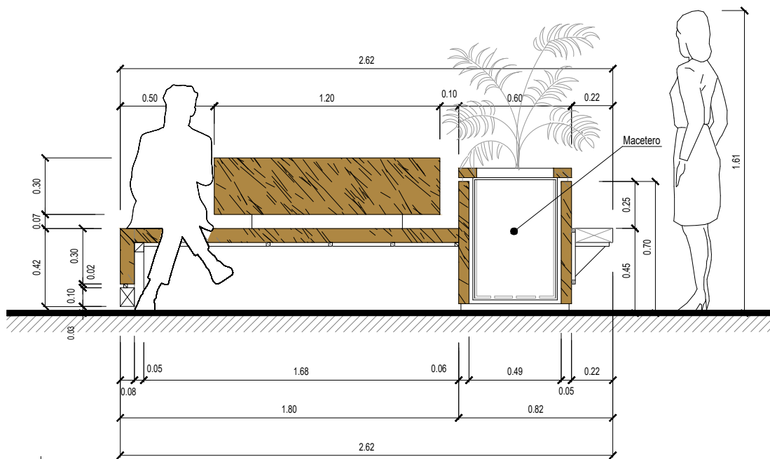
ESCAÑO N°2 CORTE LONGITUDINAL
