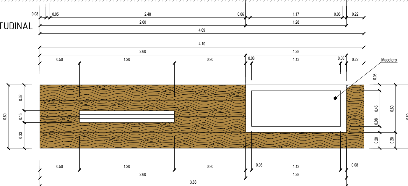
ESCAÑO N°2' PLANTA ARQUITECTURA
