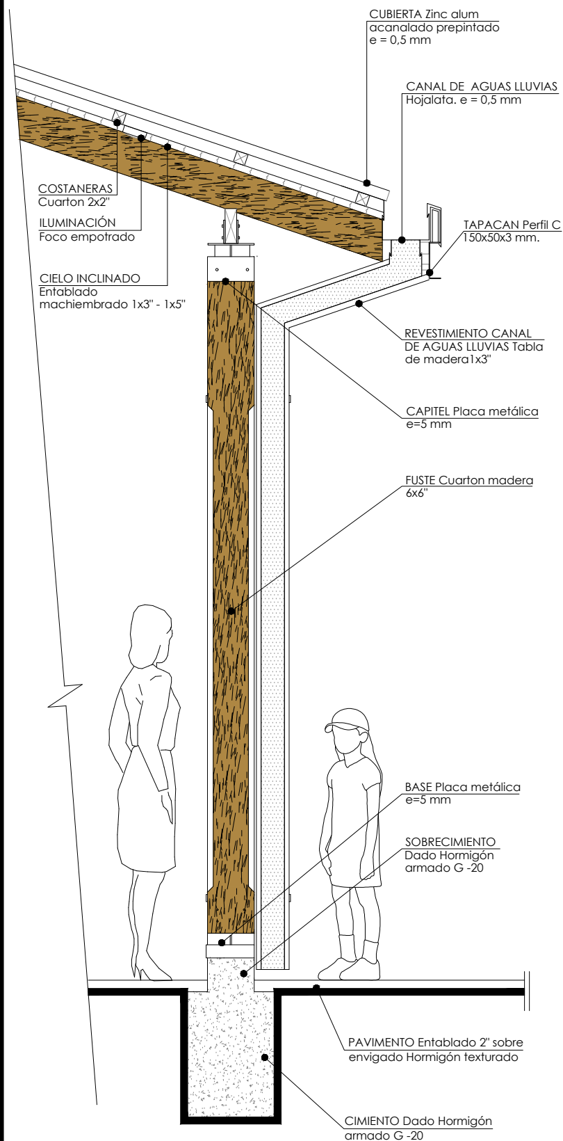
ESCANTILLON BAJADA DE AGUA Escala 1/20
