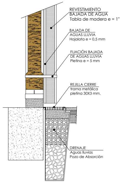
BAJADA DE AGUA Escala 1/20
