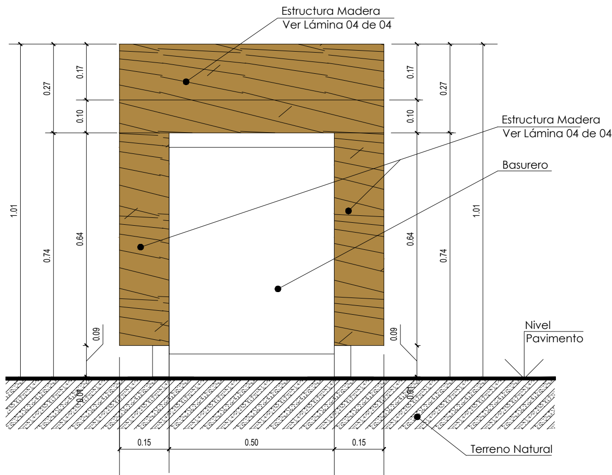
ELEVACIÓN POSTERIOR BASURERO
