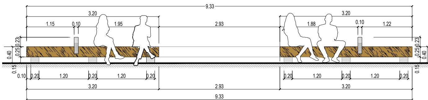
ESCAÑO N°7 ALZADO LATERAL
