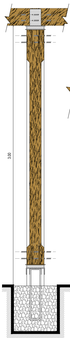
Pilar macizo N°2 Escala 1/20
