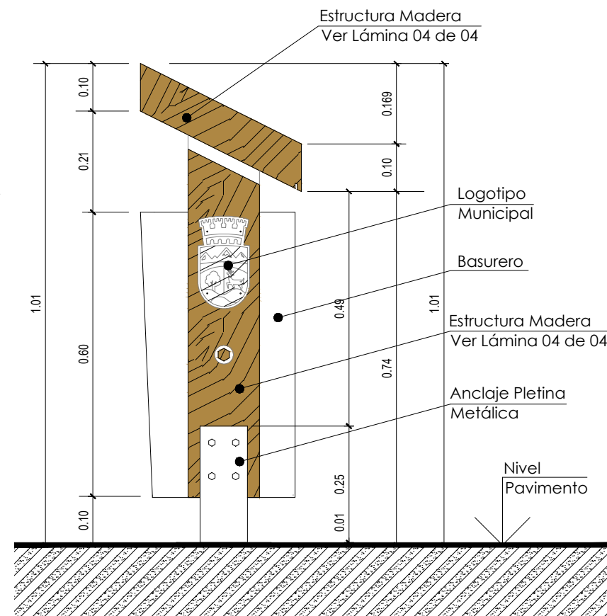
ELEVACIÓN LATERAL BASURERO
