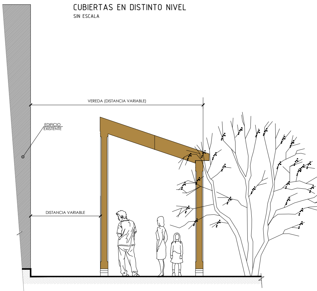
DETALLE VEREDAS CUBIERTAS DISTANCIADO DE ARBOLADO Y EDIFICIO QUE SIRVE SIN ESCALA
