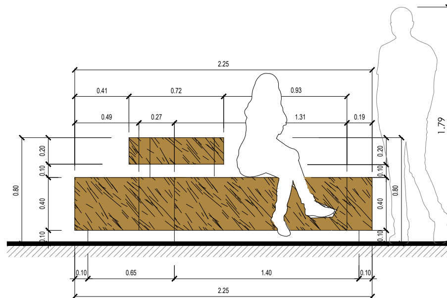
ESCAÑO N°3 ALZADO FRONTAL
