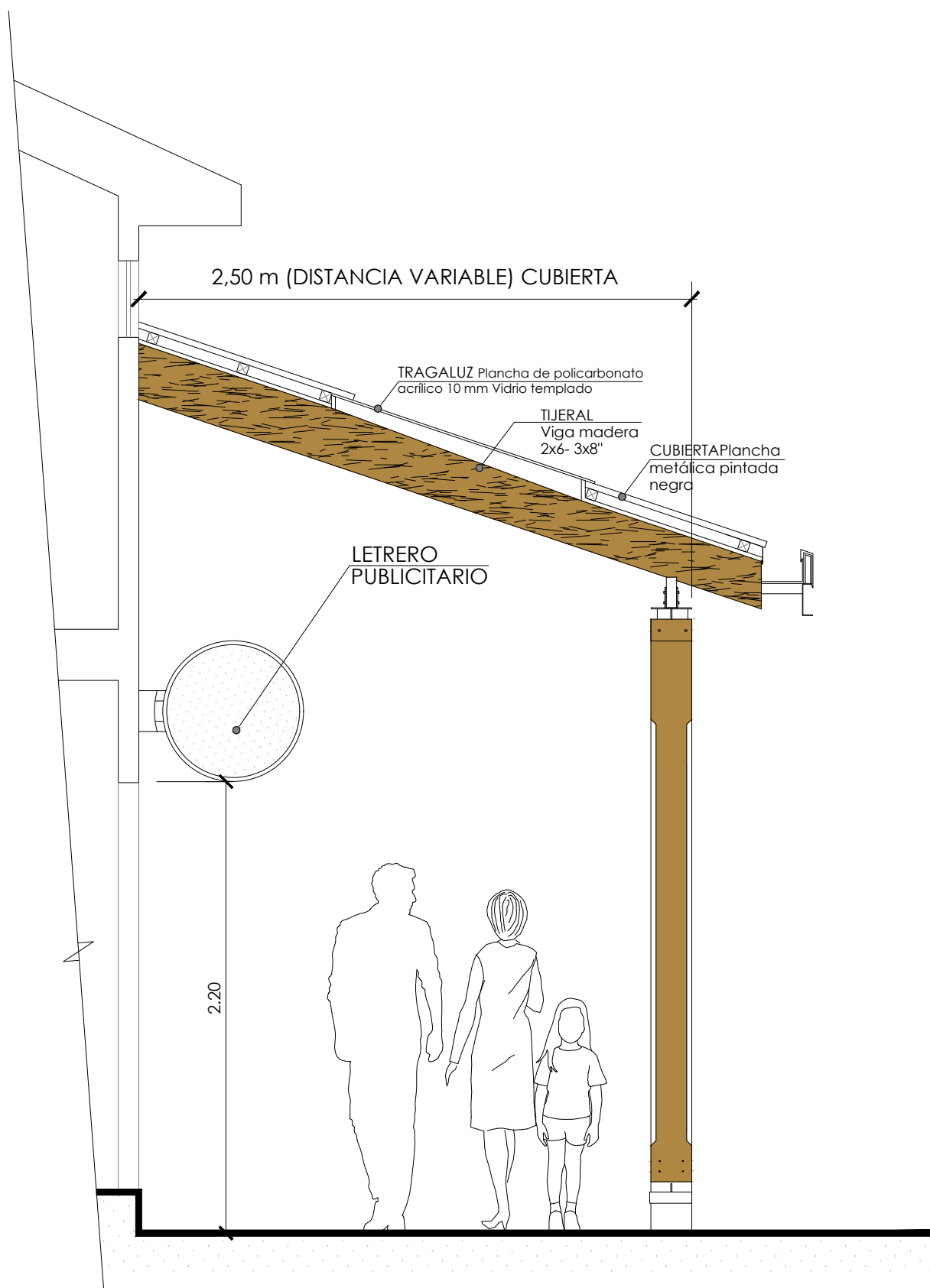
DETALLE TRAGALUZ VEREDA CUBIERTA
