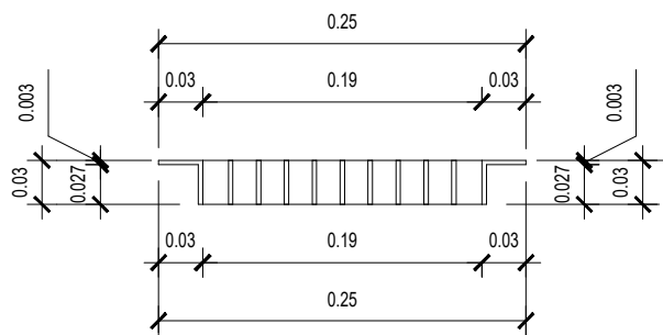
CORTE REJILLA
