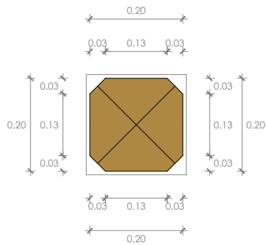
Planta Pilar macizo
