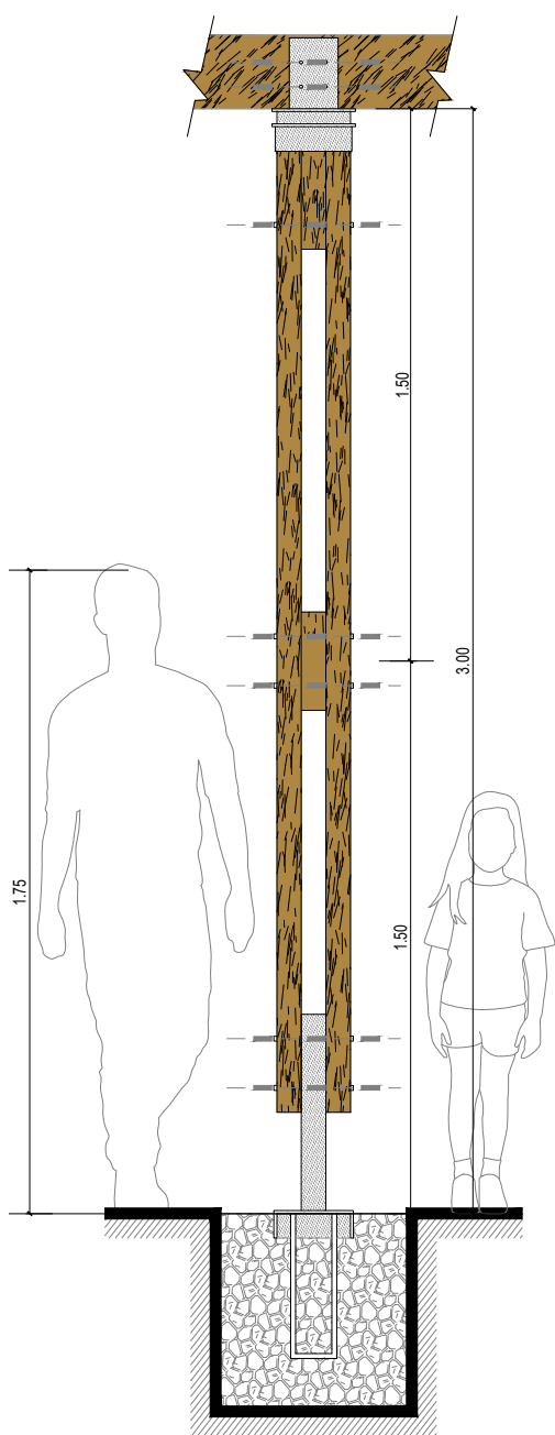
Pilar armado N°1 Escala 1/20
