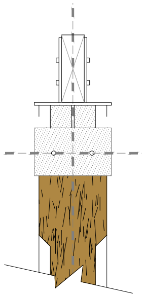
Alzado lateral capitel alternativa 2
