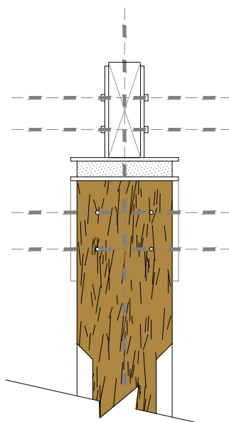
Alzado lateral. Capitel Alternativa N°1. Escala 1/10
