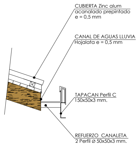
CORTE REJILLA Escala 1/20
