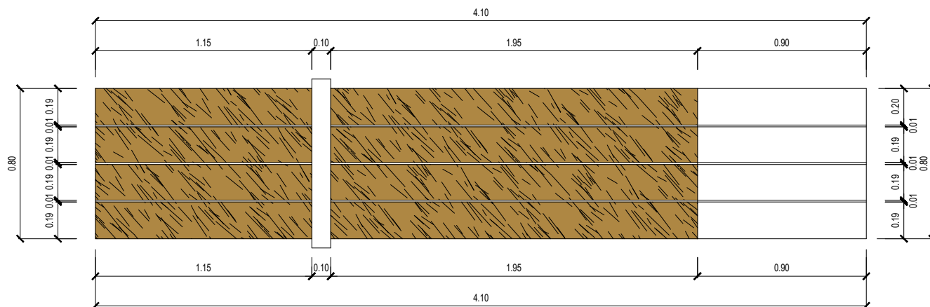
ESCAÑO N°5 PLANTA DE ARQUITECTURA
