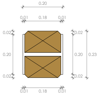
Planta Pilar metálico revestido 1
