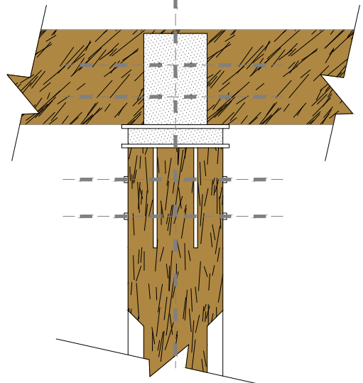
Alzado frontal capitel alternativa 4
