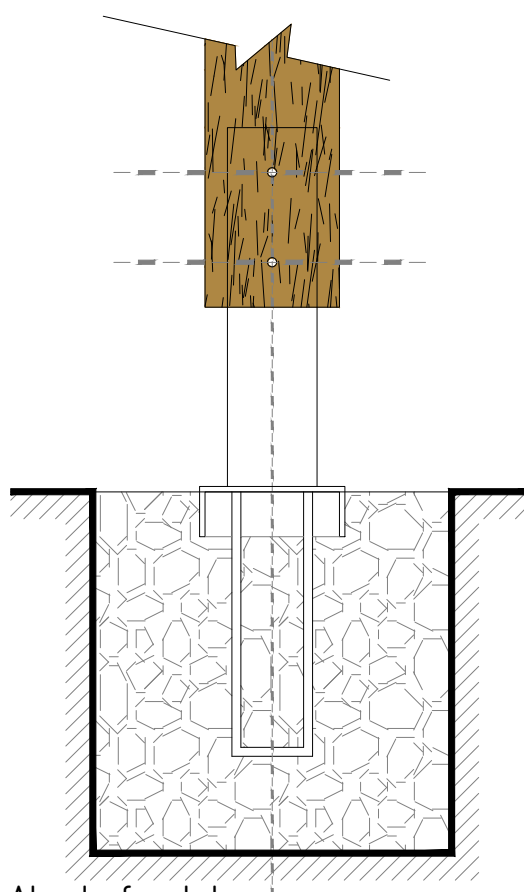
Alzado frontal Base alternativa 3
