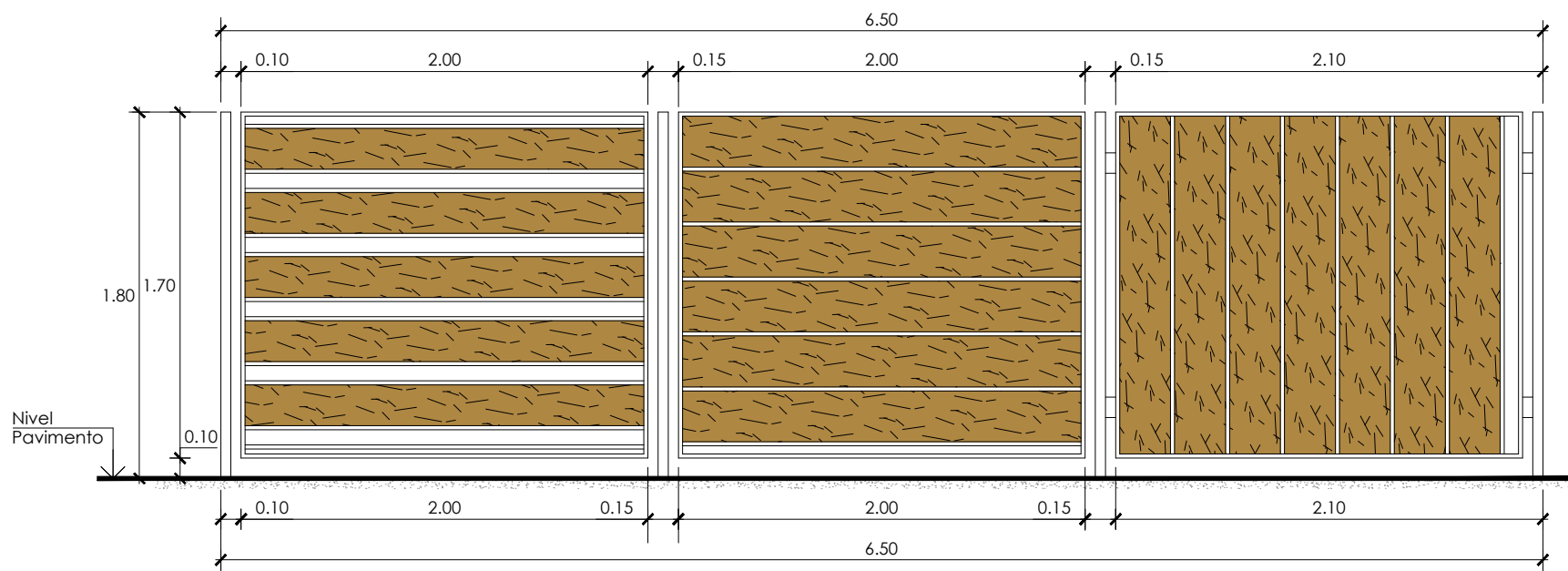
CIERRO PERIMETRAL ALTERNATIVA 4 ESCALA 1/30
