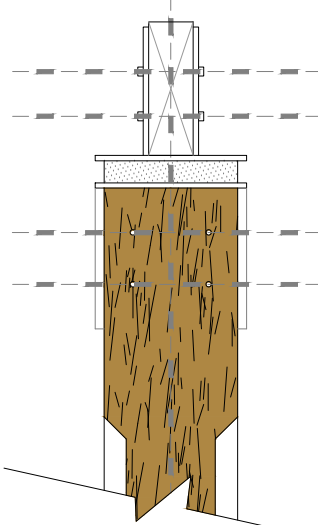
Alzado lateral capitel alternativa 4
