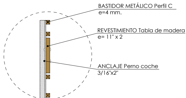
DETALLE ALTERNATIVA 3 ESCALA 1/5
