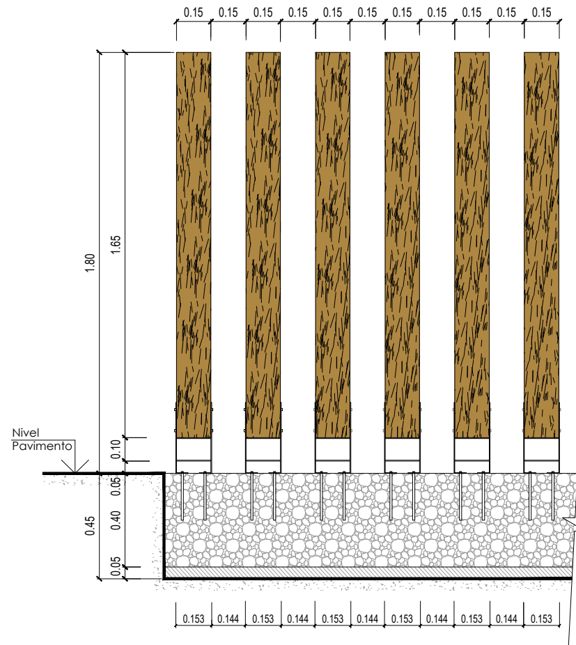
CIERRO PERIMETRAL ALTERNATIVA 1
