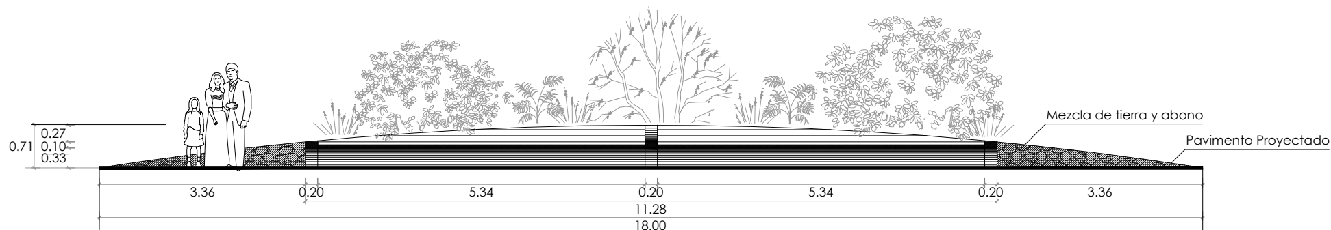
ALZADO FRONTAL ESCALA 1/75
