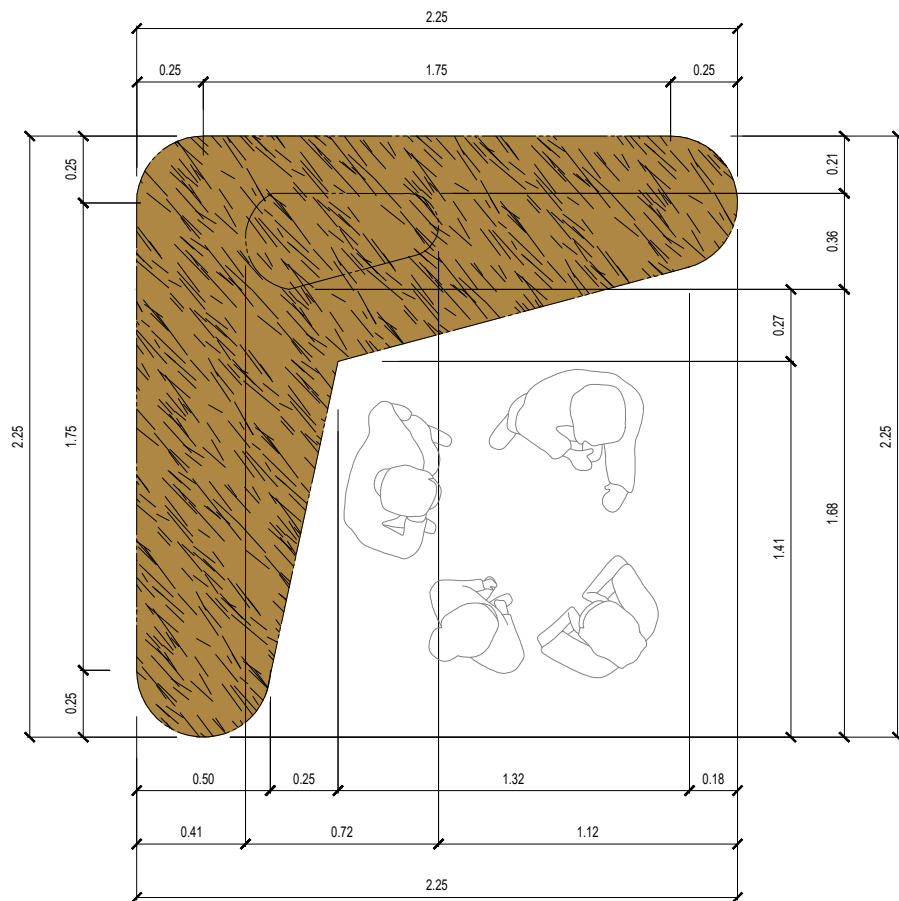
ESCAÑO N°3 PLANTA DE ARQUITECTURA
