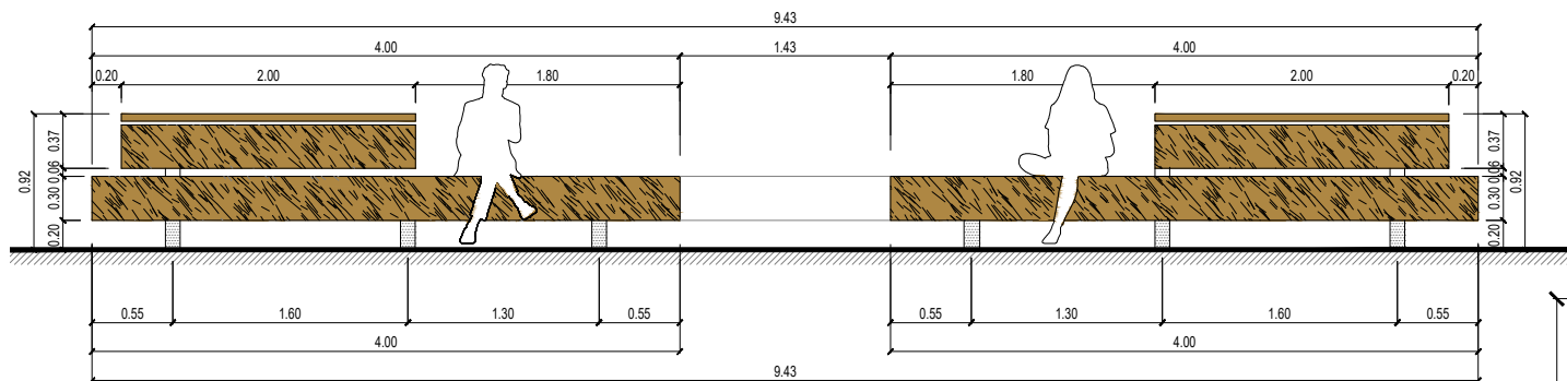
ESCAÑO N°1 ALZADO FRONTAL
