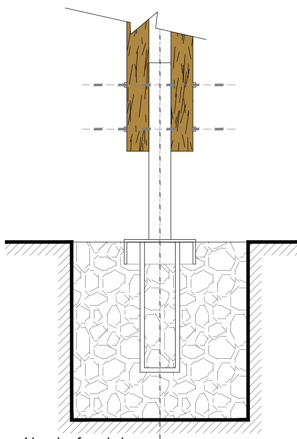
Alzado frontal Base alternativa 4
