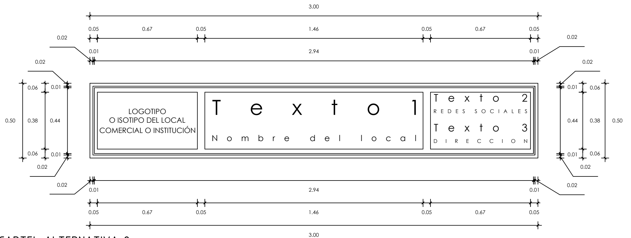
CARTEL ALTERNATIVA 2 ESCALA 1/20
