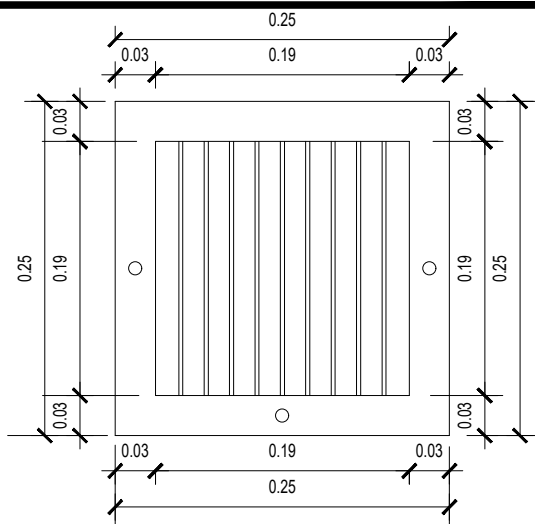
PLANTA REJILLA
