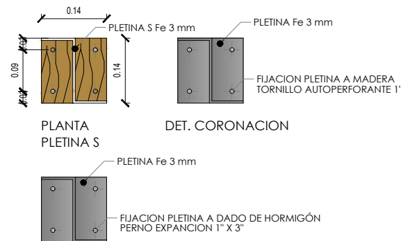
DET. FIJACION AL PISO
