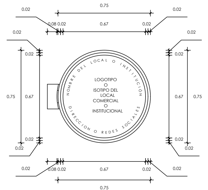
CARTEL ALTERNATIVA 4 ESCALA 1/20
