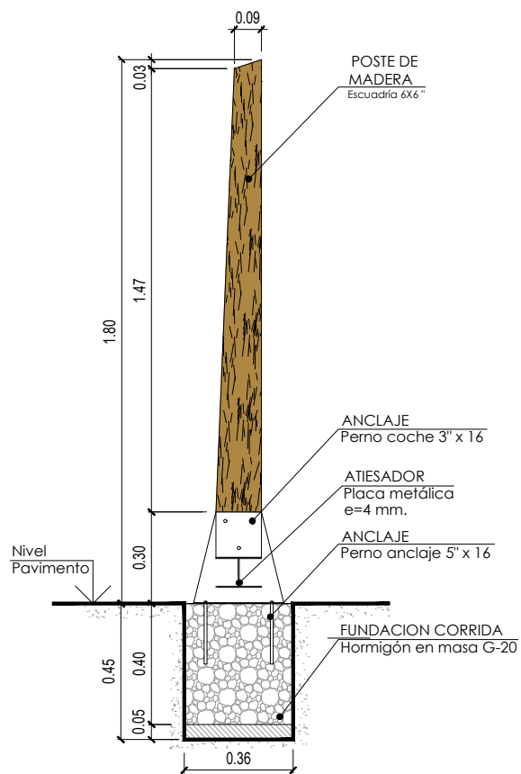
CORTE TRANSVERSAL ALTERNATIVA 1
