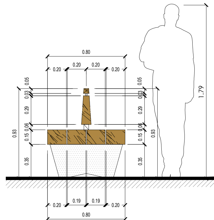
ESCAÑO N°4 CORTE TRANSVERSAL
