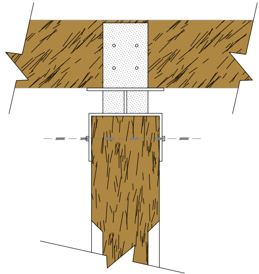
Alzado frontal capitel alternativa 2
