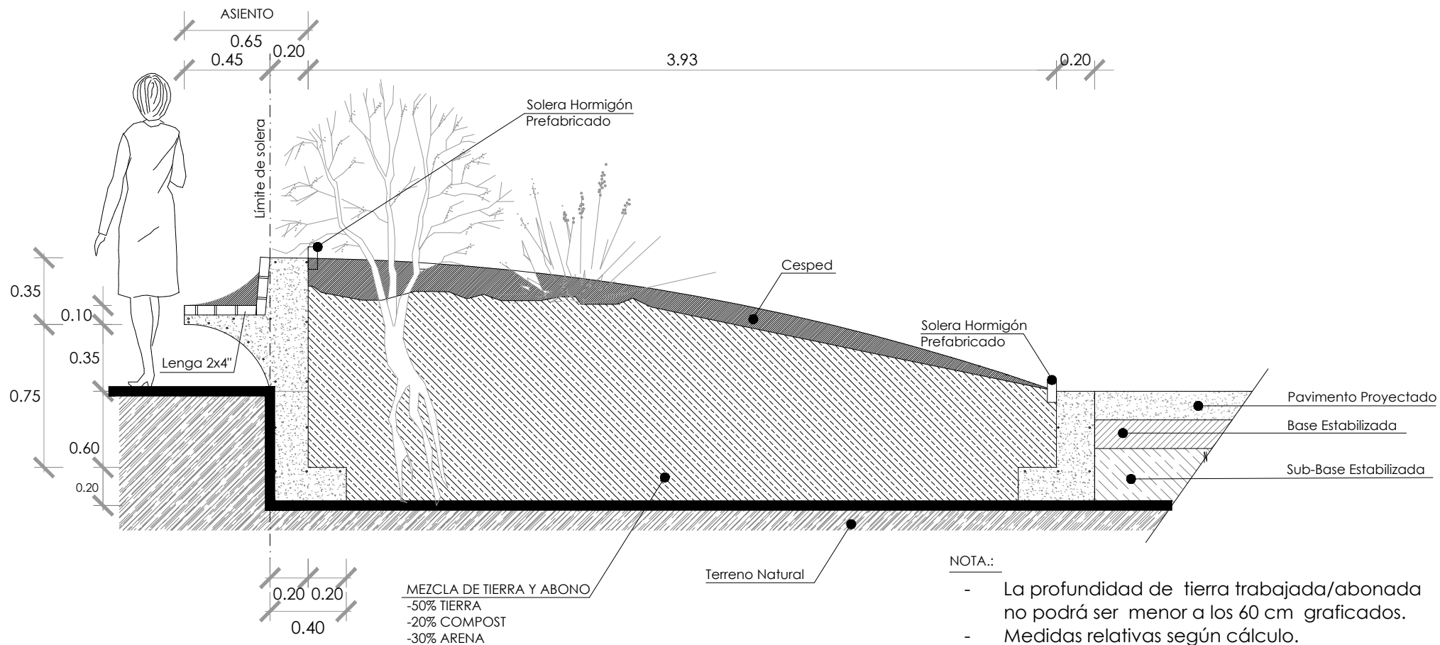
CORTE TRANSVERSAL TÚMULO ESCALA 1/25
