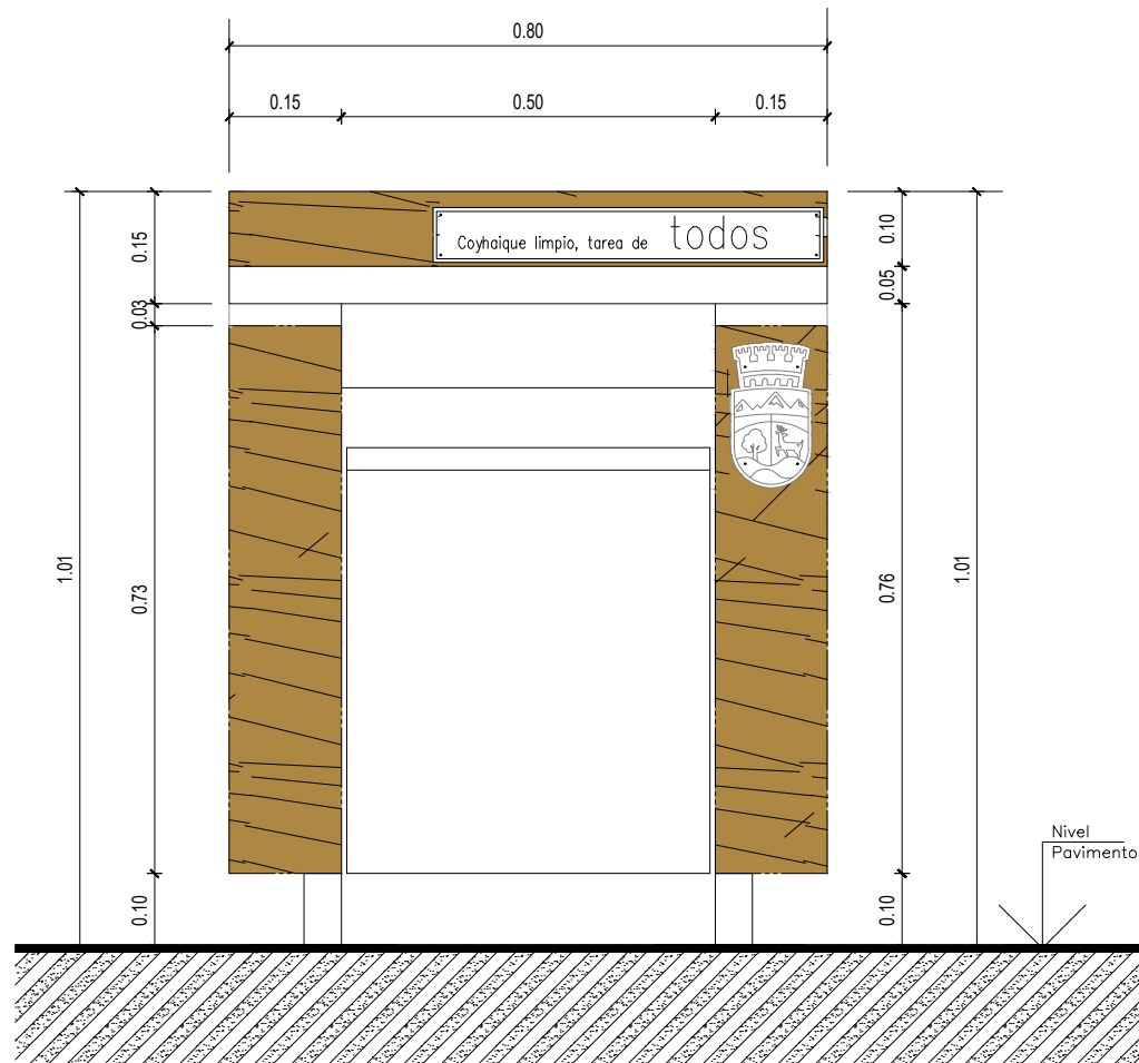
ELEVACIÓN FRONTAL BASURERO
