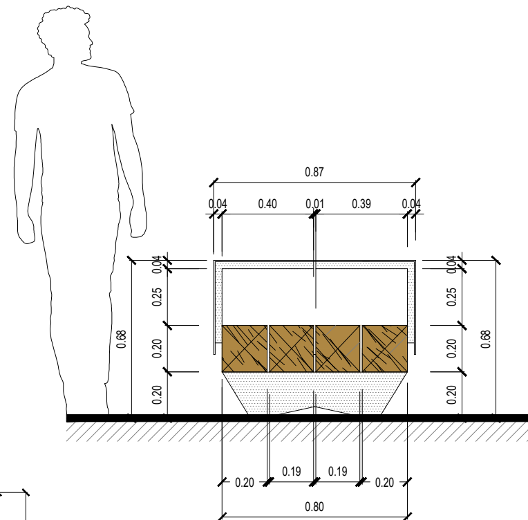
ESCAÑO N°5 CORTE TRANSVERSAL
