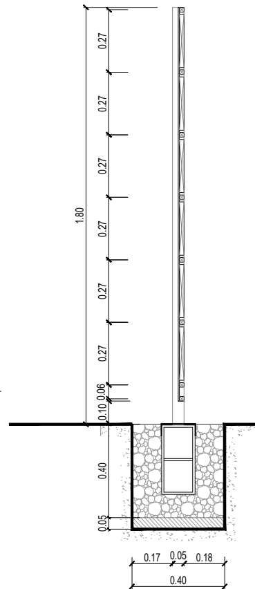
CORTE TRANSVERSAL ALTERNATIVA 4
