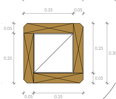
Planta Pilar metálico revestido 2
