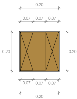
Planta Pilar armado alternativa 2
