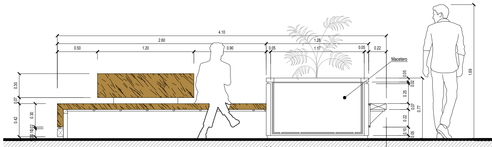
ESCAÑO N°2' CORTE LONGITUDINAL
